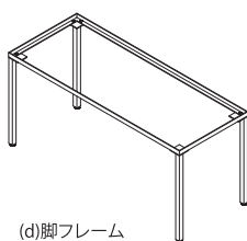
(d)脚フレーム H:700 W:1500 D:600 クロームメッキ
