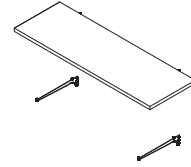
(d) 棚板(受金具セット) W:1200 D:400 t:25 天面:化粧合板(白) 見付:木口テープ(木目) 照明:ラインLED N1200内蔵 消費電力:16.2W
