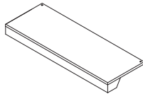
(e) 棚受金具(ガラス棚、傾斜棚) H:86 W:900 D:417 クロームメッキ 照明:ラインLED N900内蔵 消費電力:10.8W
