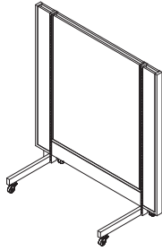
(a) 本体 H:1350 W:1200 D:560~850 スチールフレーム:粉体塗装仕上 パネル:リバーシブル化粧合板(木目、白)
