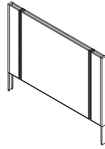
(b) 本体 H:950 W:1200 D:50 スチールフレーム:粉体塗装仕上 パネル:リバーシブル化粧合板(木目、白)
