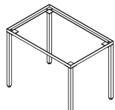
(b)-2脚フレーム H:700 W:900 D:600 クロームメッキ
