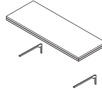
(k) バラベット H:50 W:1200 D:450 底面/天面:化粧合板(白) 見付:木口テープ(木目) 照明:ラインLED N1200内蔵 消費電力:16.2W 受金具:シロアゲ
